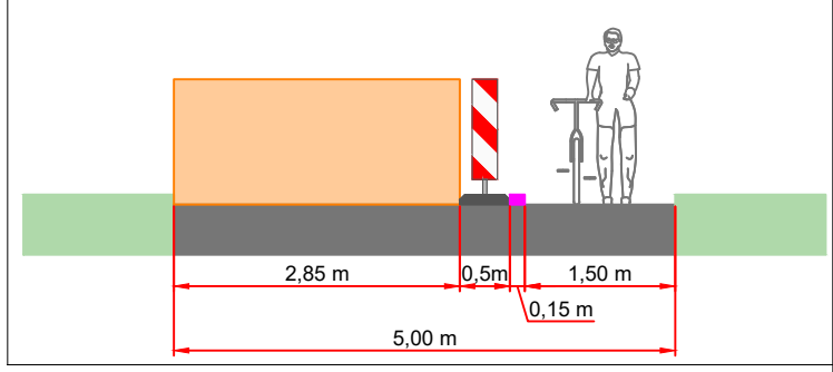
Dwarsdoorsnede A-A
