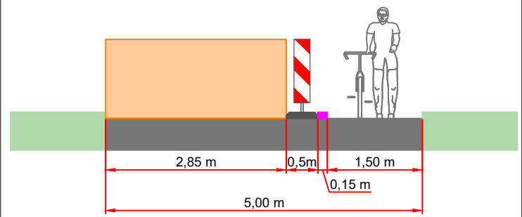
Dwarsdoorsnede A-A
